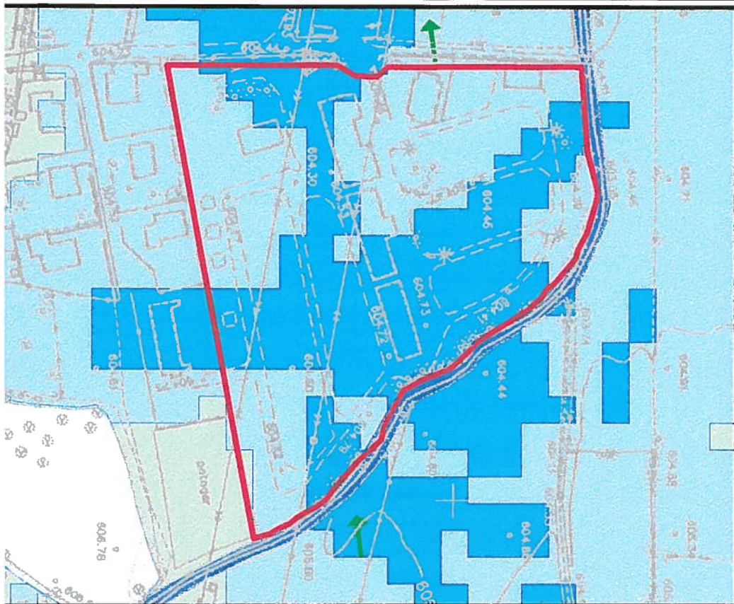
Carte des hauteurs d'eau et des vitesses pour une crue type 1925
