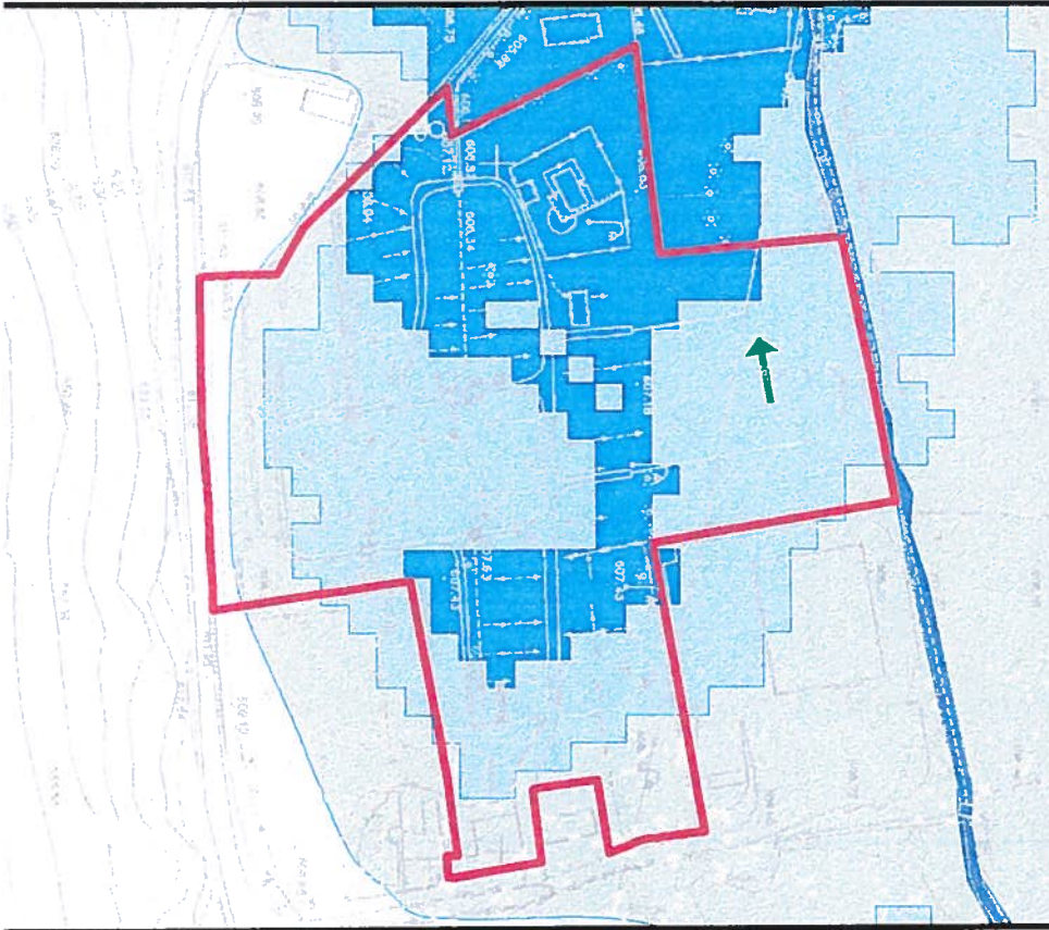
Carte des hauteurs d'eau et des vitesses pour une crue type 1925
