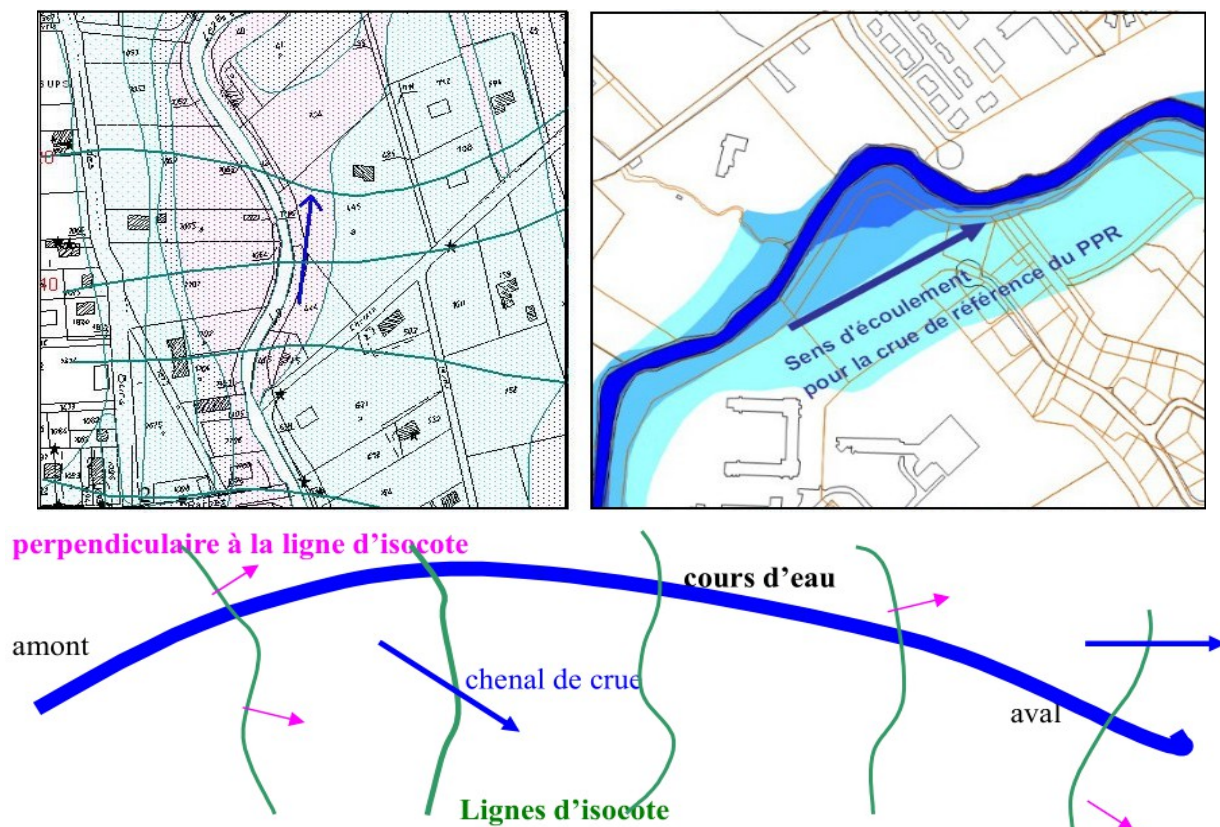
Sens d'écoulement des eaux : emprise de la ligne d'eau selon l'angle du bâtiment (exemples)
