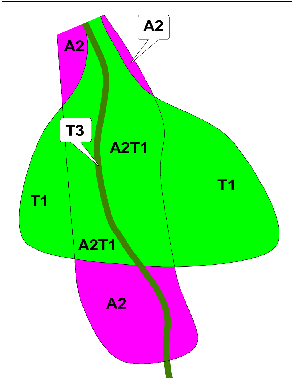
Figure n°5 : Principe de cartographie des aléas
