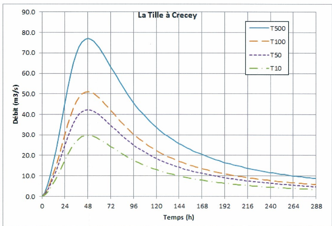
Figure 10 : Hydrogrammes synthétiques – Station de Crecey-sur-Tille
