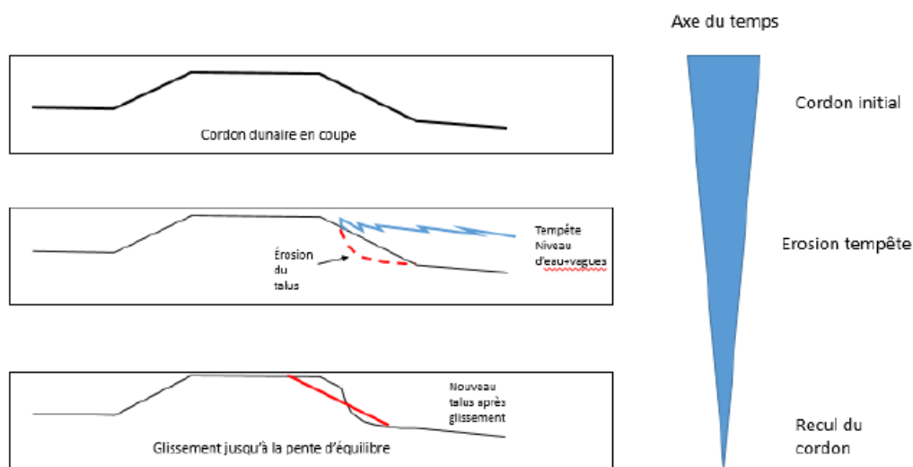
Schématisation du recul par érosion du cordon dunaire
