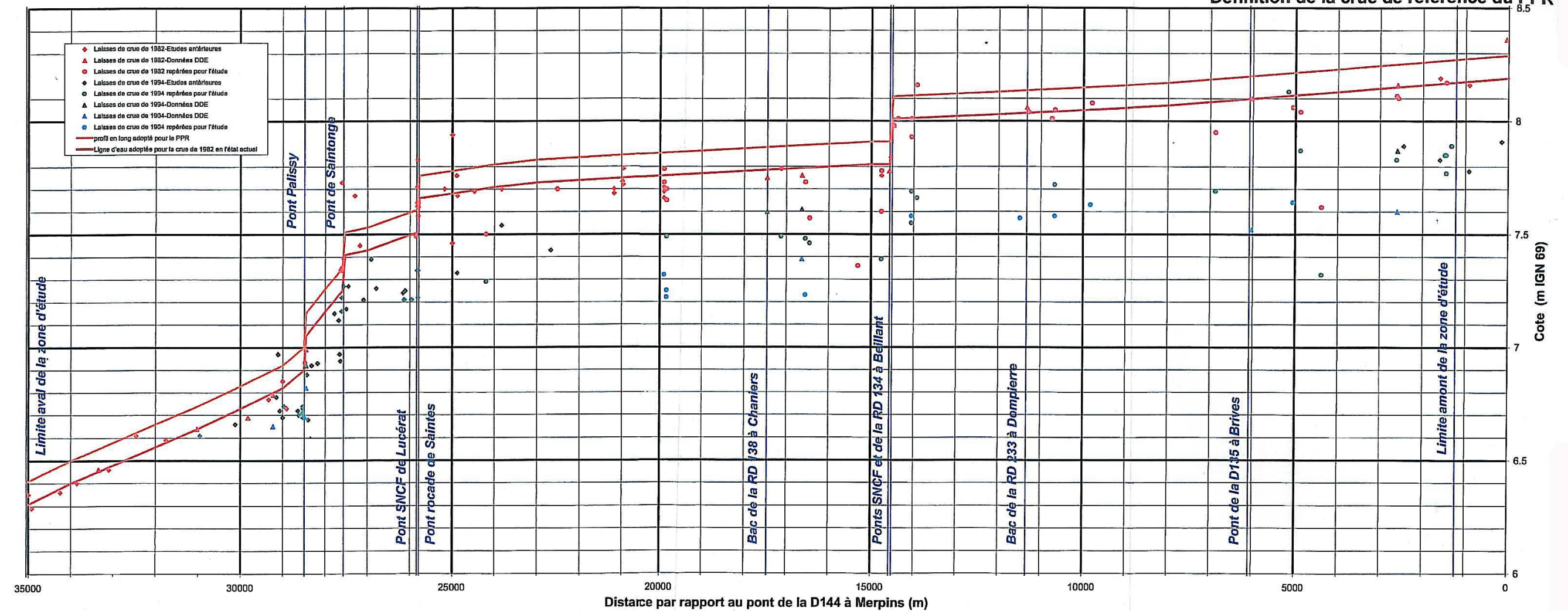
Figure 3 - 3 Profil en long de la Charente Définition de la crue de référence du PPR
