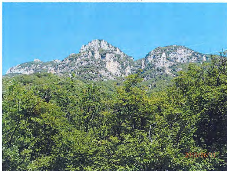
Photo n°4 : Série jurassique de la barre des Courmettes
