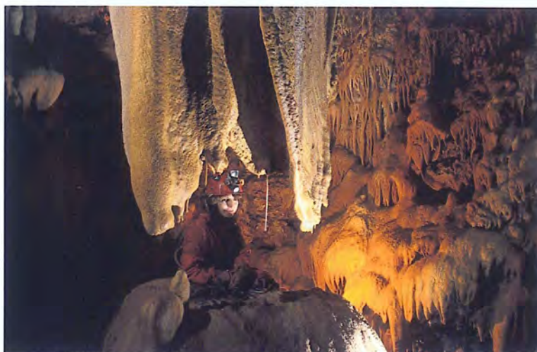
Photo n°18 : photographie de l'intérieur de l'aven Draperies
