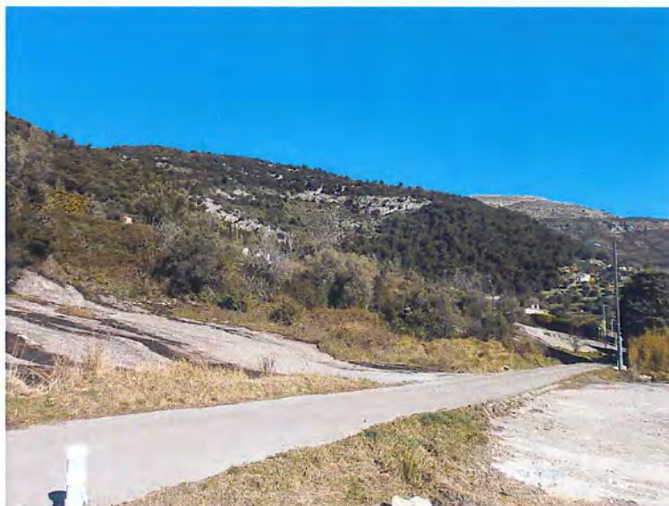
Photo n°36 : ruissellement naturel sur les dalles de molasse Quartier des Queinières
