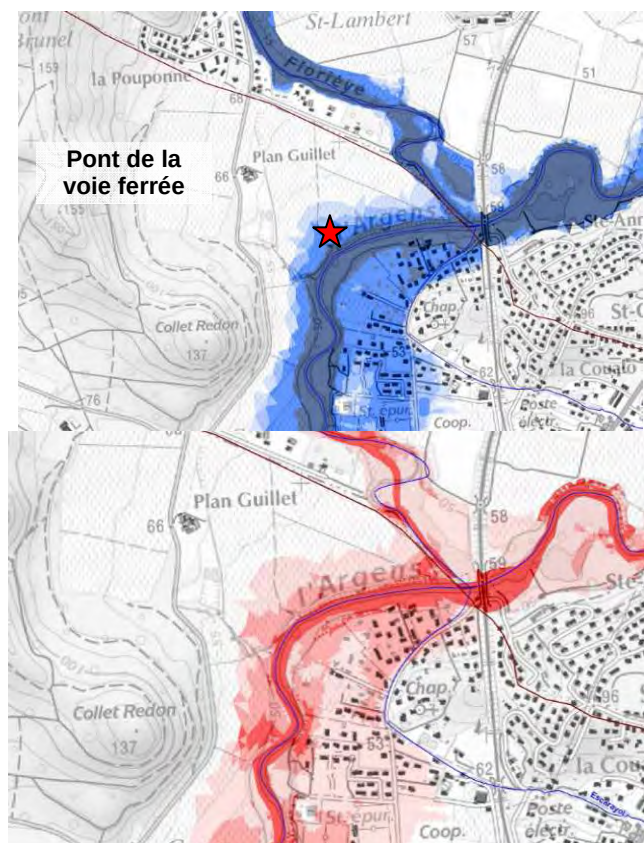
Figure 25 : Hauteur d'eau et vitesses d'écoulement – L'Argens (partie urbanisée)
