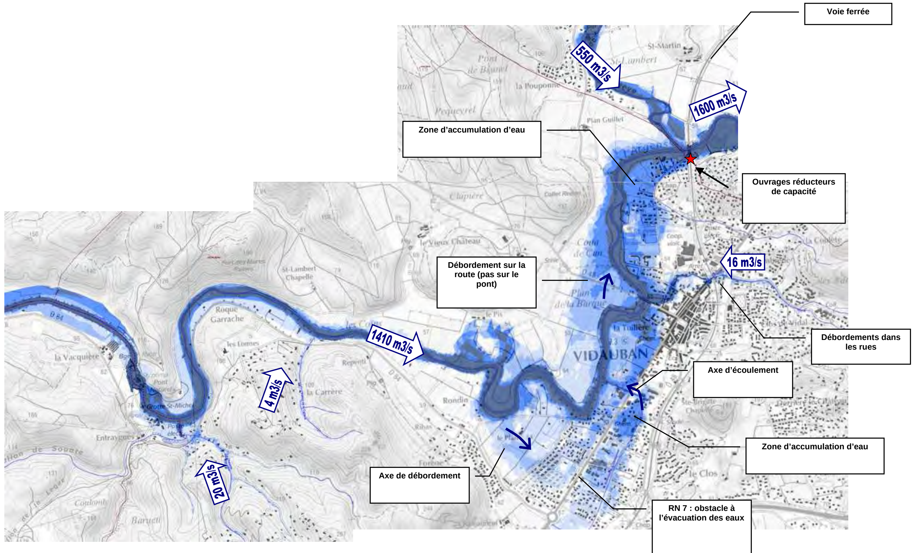
Figure 31 : Dynamique des écoulements à Viduban
