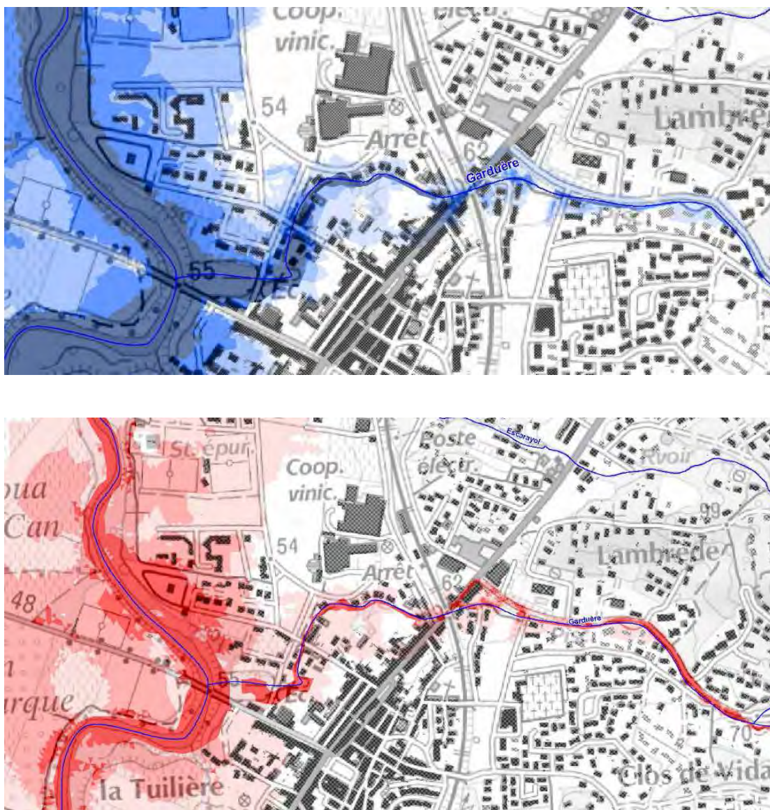
Figure 28 : Hauteur d'eau et vitesses d'écoulement – La Garduere
