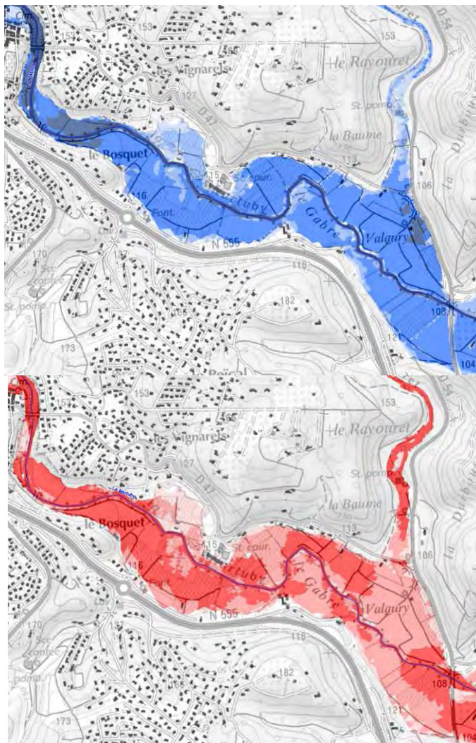
Hauteur d'eau et vitesses d'écoulement –La Nartuby en aval du village
