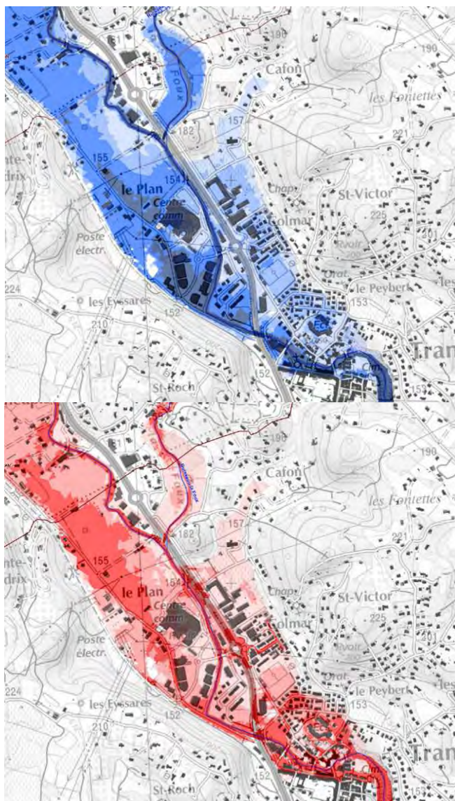
Hauteur d'eau et vitesses d'écoulement –La Nartuby en amont du village
