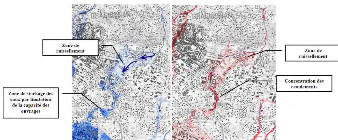
Figure 28 : Hauteur d'eau et vitesses d'écoulement – Le vallon des Tours
