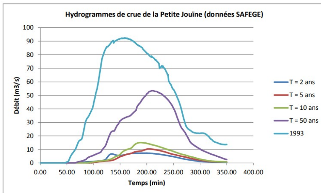
Figure 20 : Hydrogrammes de crue de la Petite Jouïne au niveau de la RD9 d'après SAFEGE (source : INGEROP – SABA, 2013)
