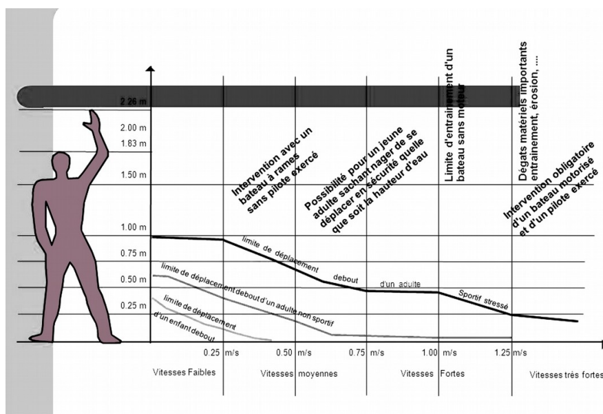
Figure 40 : Mobilité en terrain inondé en fonction de la vitesse et de la hauteur d'eau
