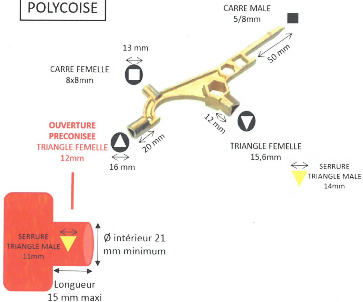
Figure 3. Caractéristiques de la clé polycoise multifonctions
