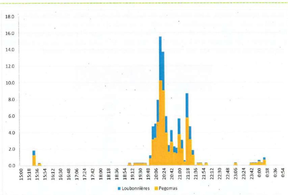
Figure 25 : Hyétogrammes du Vallon de Loubonnières et de la station de Pégomas
