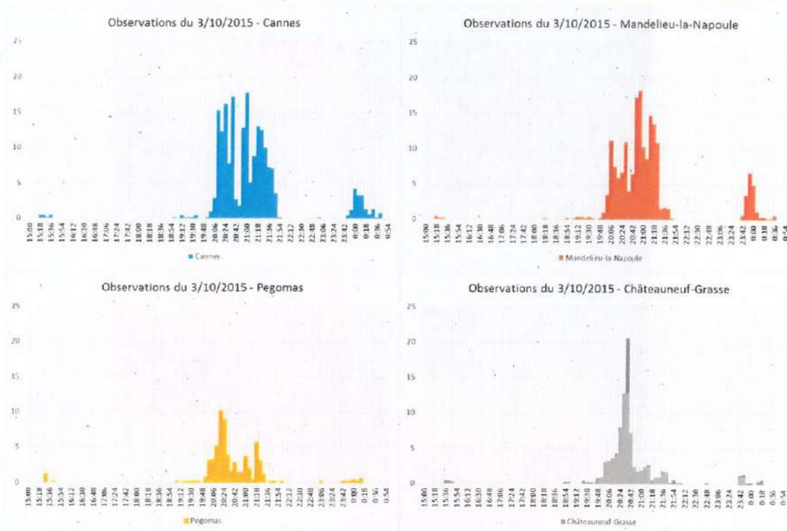
Figure 21 : Hyétoigrammes du 3 octobre 2015, centrés sur l'évènement
