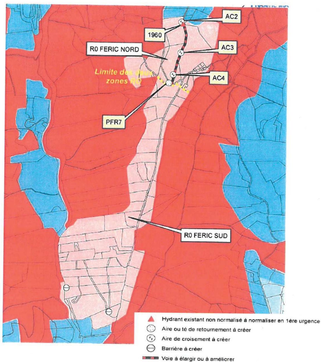
Schéma des aménagements réalisés (extrait de la carte des travaux du PPRIF approuvé en 2017)
