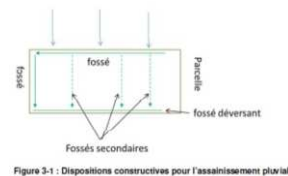
Figure 3-1 : Dispositions constructives pour l'assainissement pluvial
