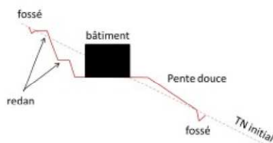
Figure 3-3 : Dispositions constructives pour les déblais remblais
