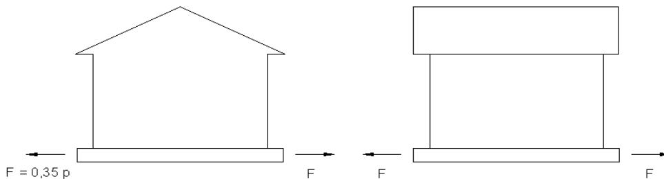
Efforts horizontaux dans les fondations
