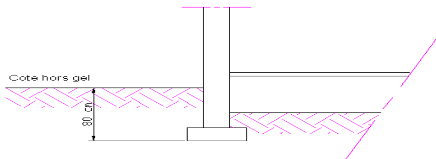
Profondeur d'ancrage des fondations
