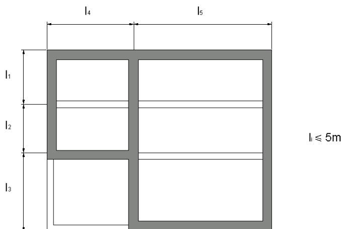
Maillage des fondations
