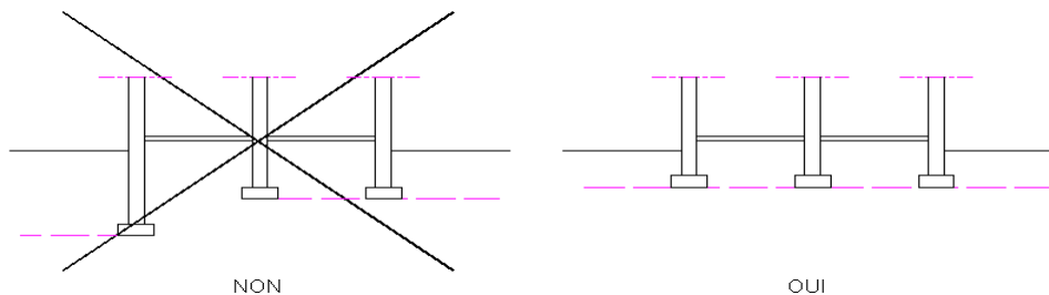
Plan d'assise des fondations
