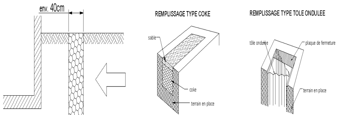
Exemple de tranchée compressible périphérique
