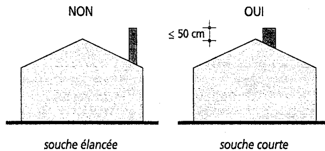
Conduits de fumée.
