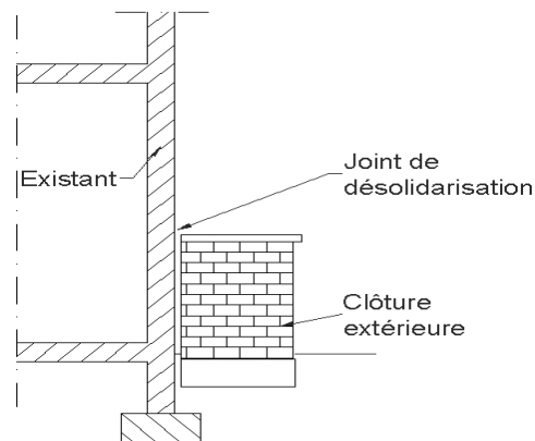
Désolidarisation des ouvrages secondaires
