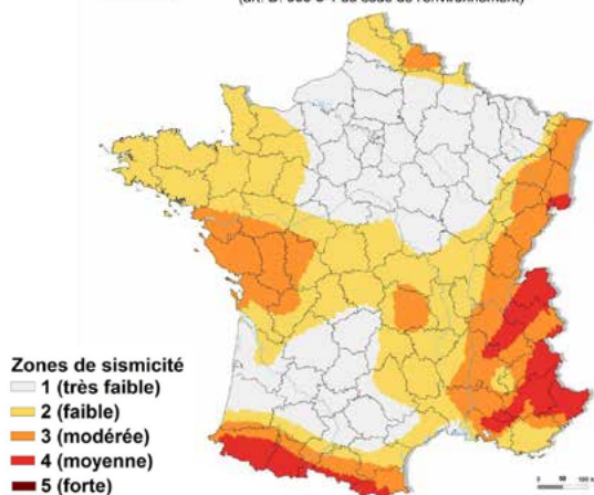
Zonage sismique de la France en vigueur depuis le 1er mai 2011 (art. D. 563-8-1 du code de l'environnement)
