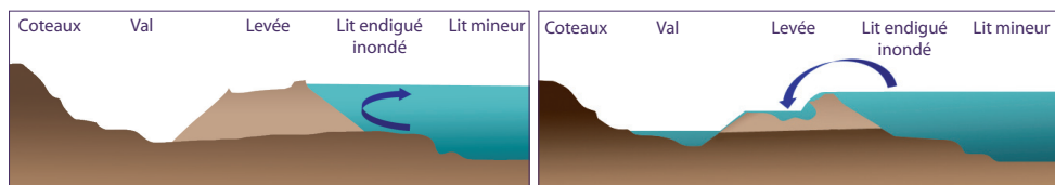
1. Rupture d'ensemble d'une levée due à de fortes pressions et à une fragilité de l'ouvrage
