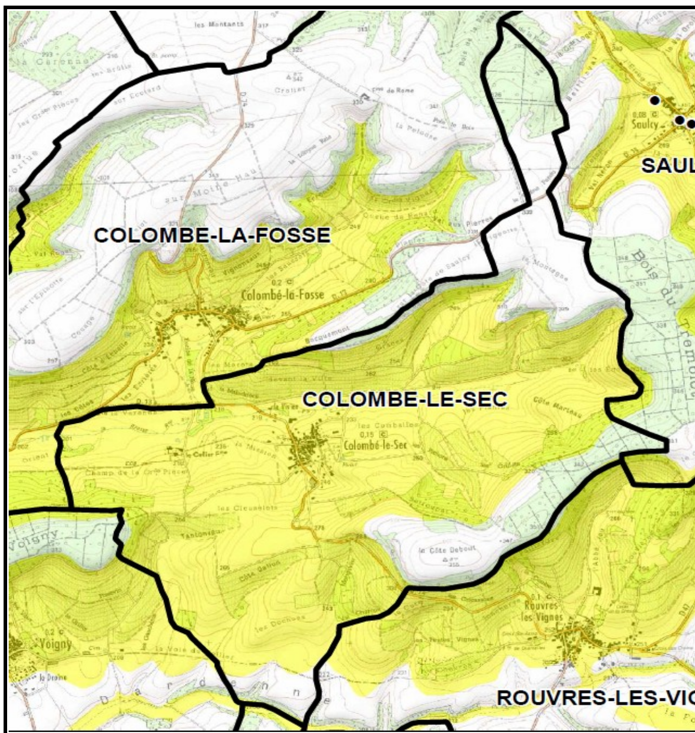
Carte des zones susceptibles de présenter un risque de mouvement de terrain sur la commune de Colombé-le-Sec
